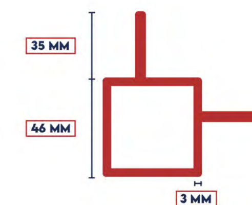
CONNECTEUR DE COIN
